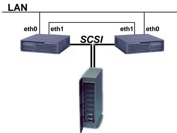
FIG. 1: struttura del cluster usato per i servizi di posta elettronica e web prima della ristrutturazione.
