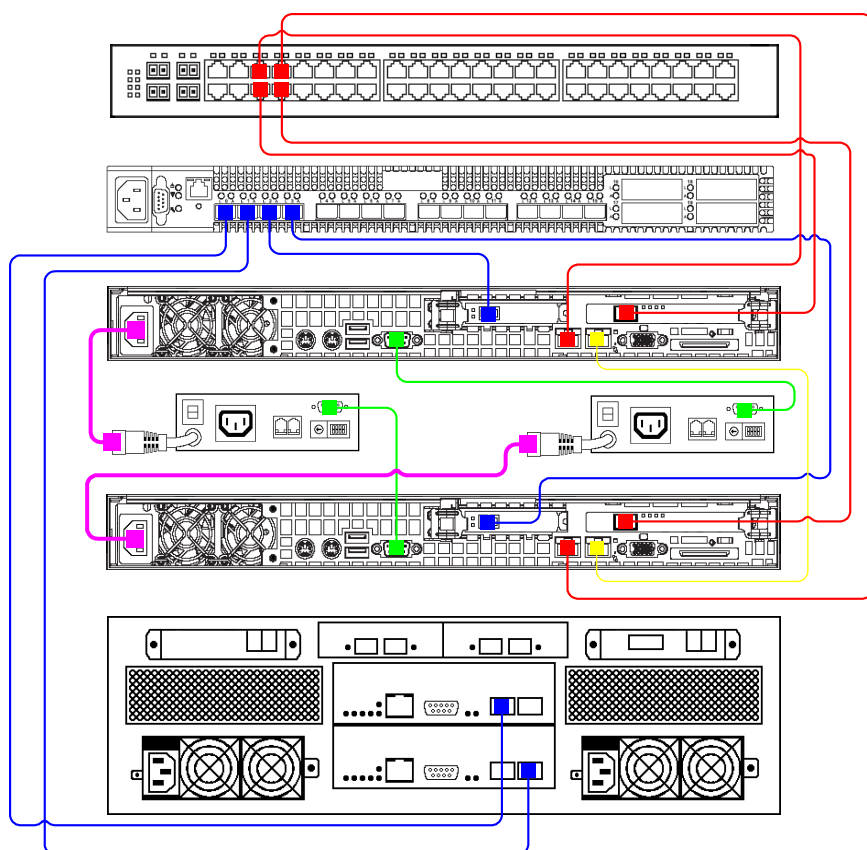
FIG. 3: schema di collegamento.
